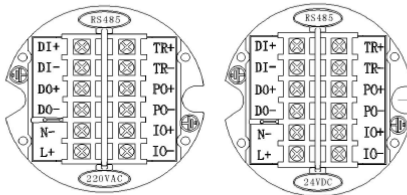
Fig. 1.2 Diagrama dos terminais de ligação
